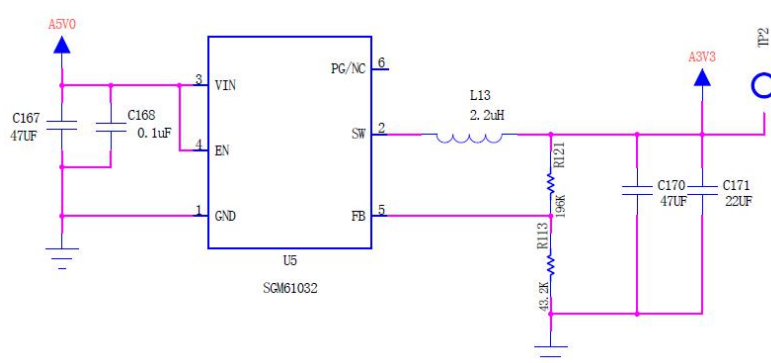
图 3-14 5V 转 3.3V 原理图
