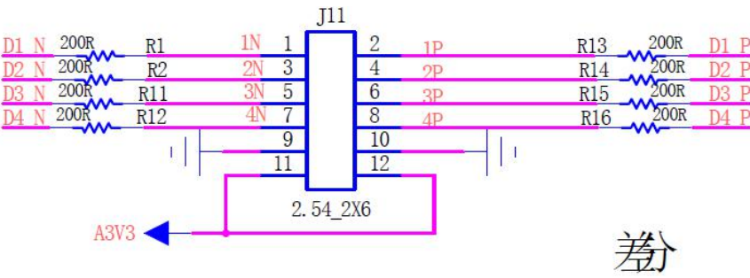
图 3-12 PMOD 座连接原理图
