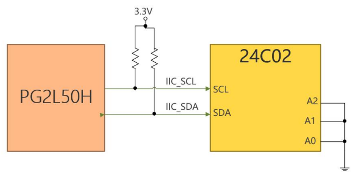
图 3-10 EEPROM 设计示意图
