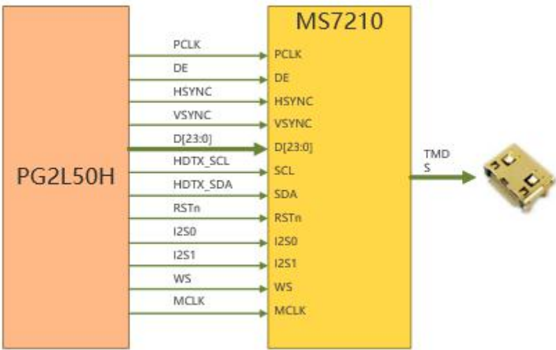
图 3-7 HDMI Transmit 连接示意图
