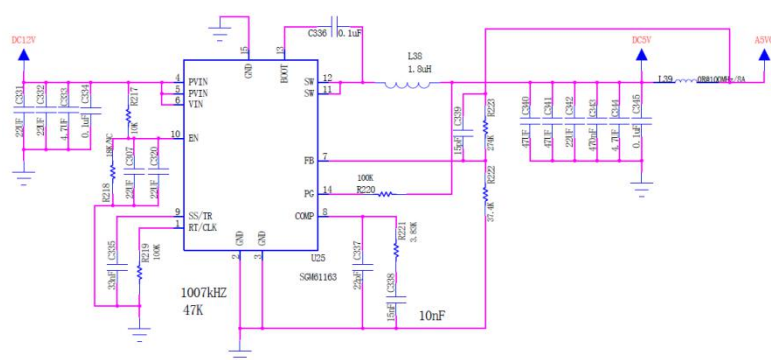
图 3-13 12V 转 5V 原理图
