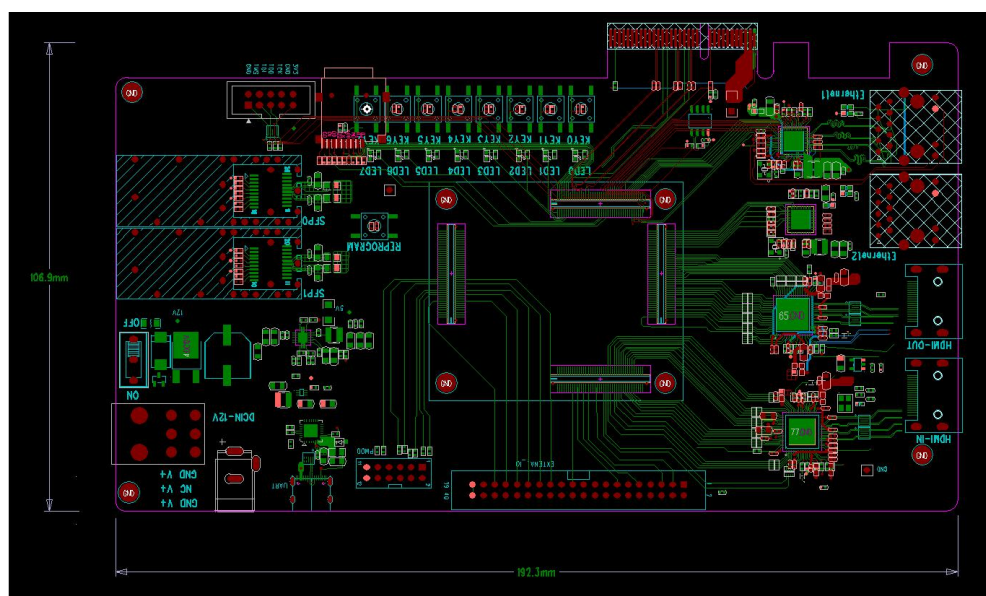
图 3-15 扩展底板尺寸结构图
