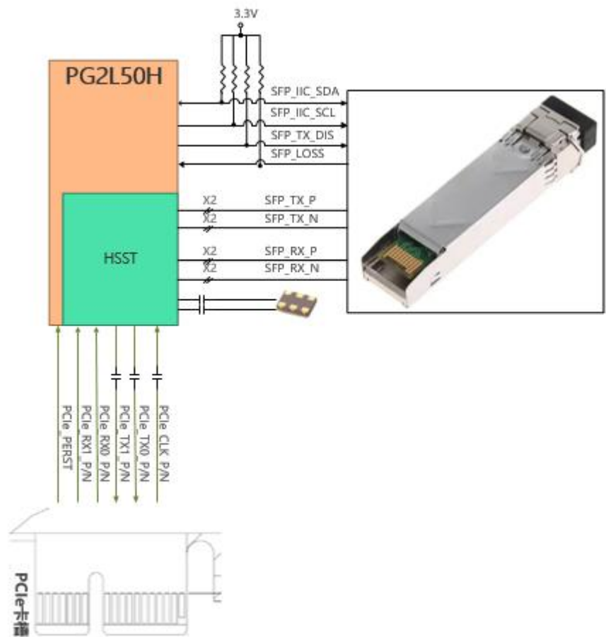
图 3-2 PG2L50H HSST 功能连接图
