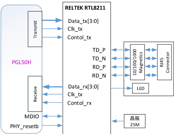
图 3-1 RTL8211 连接示例
