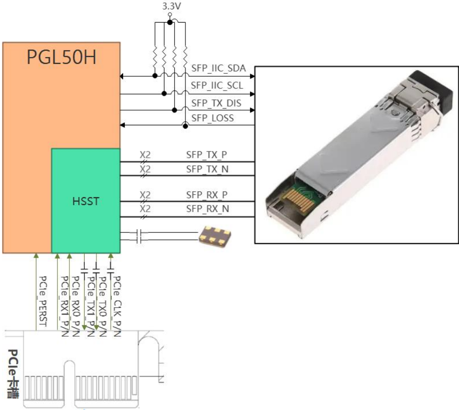
图 3-2 PGL50H HSST 功能连接图
