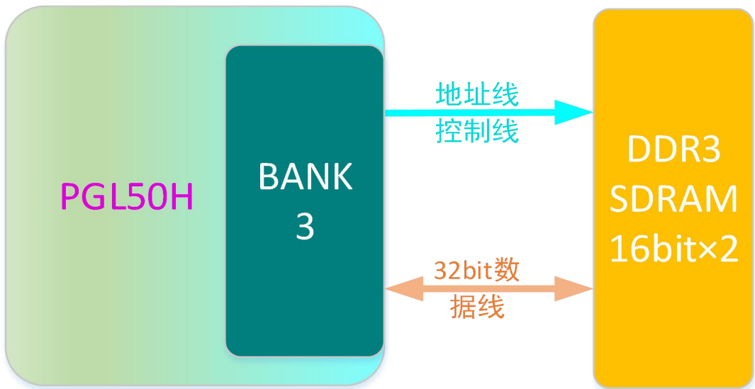
图 2-5 PGL50H 与 DDR 连接框图
