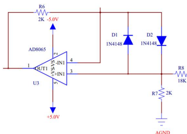
图 9 衰减电路
